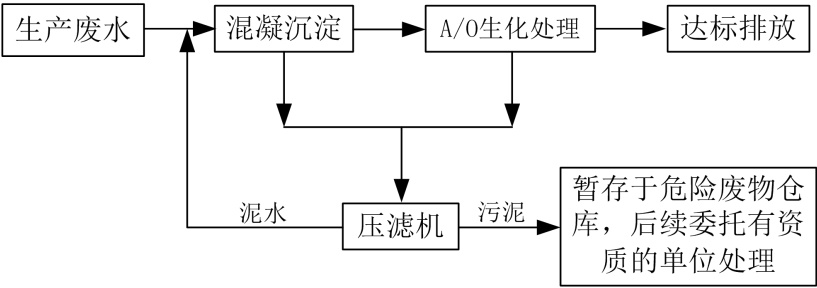
图 4.2-1 生产废水处理工艺流程图
